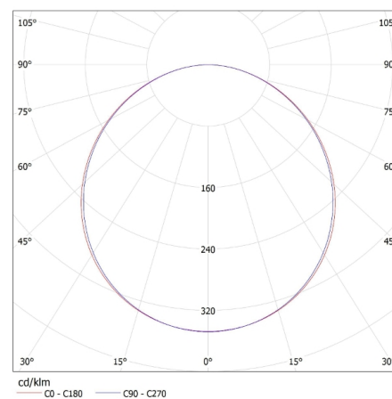
MILEDO (kat 31132) BAREV LED N 45W-NW / LDC (Polar)
