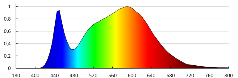
MILEDO (kat 31132) BAREV LED N 45W-NW / LDC (Polar)
